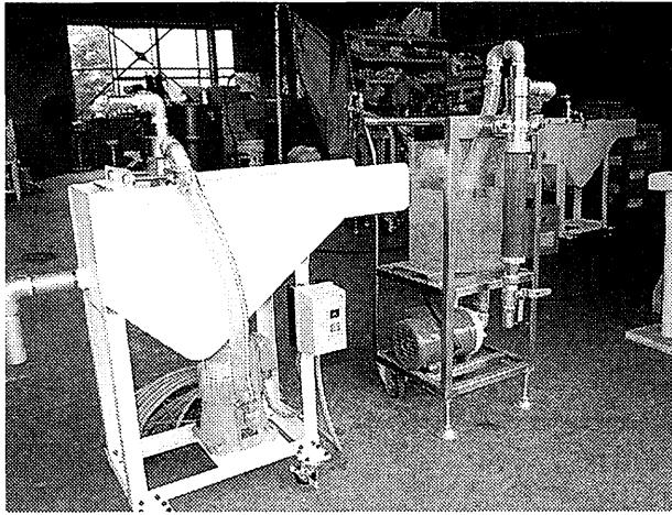
ギャザータンクキット(左)とデモ機
